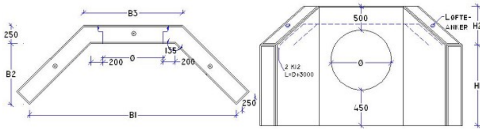
TEGNINGEN VISER TILSLUTNING MED HUFFE. ANGIV TILSLUTNINGSTYPE SPIDSBENDE ELLER HUFFE VED BESTILLING.
